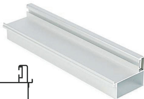
B-04 Bočni profil Side Strut Profile (beside) Боковой Профиль
